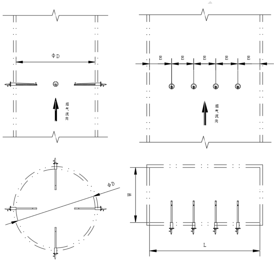
图 1 圆形烟道内单层喷枪的布置示意图
